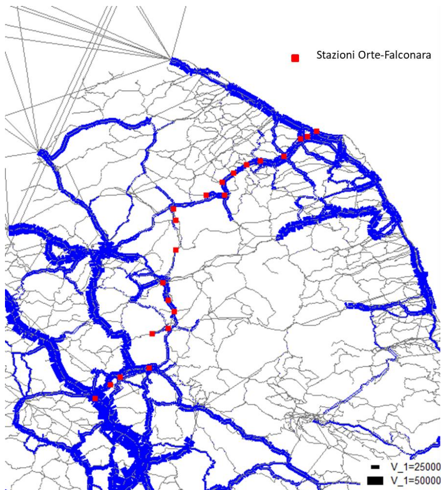
Figura 24 - Flussogrammi auto (veicoli/g), scenario progetto 2035
