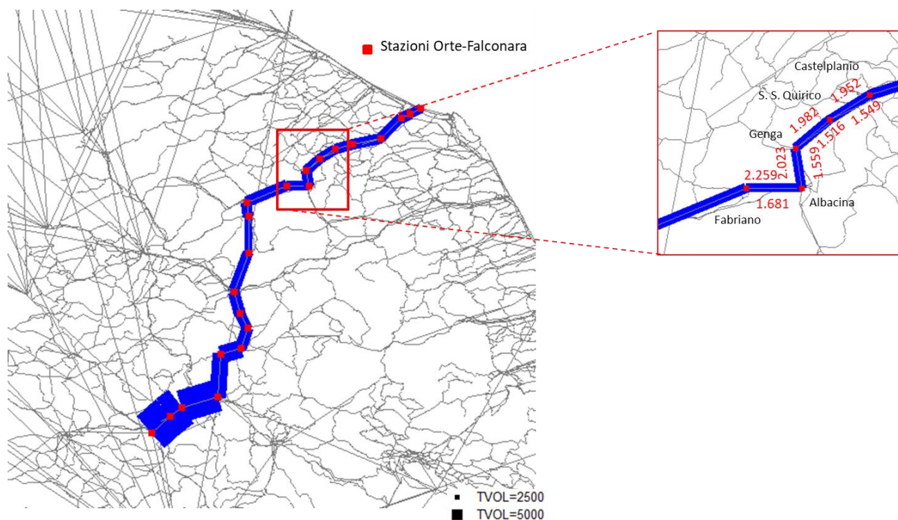
Figura 22 - Flussogrammi trasporto ferroviario (pax/g) linea Orte-Falconara, scenario di progetto 2032
