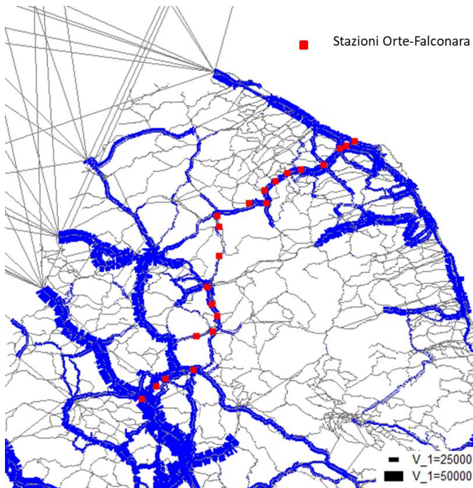
Figura 31 - Flussogrammi auto (veicoli/g), scenario riferimento 2064
