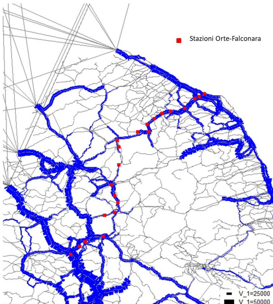
Figura 28 - Flussogrammi auto (veicoli/g), scenario progetto 2040
