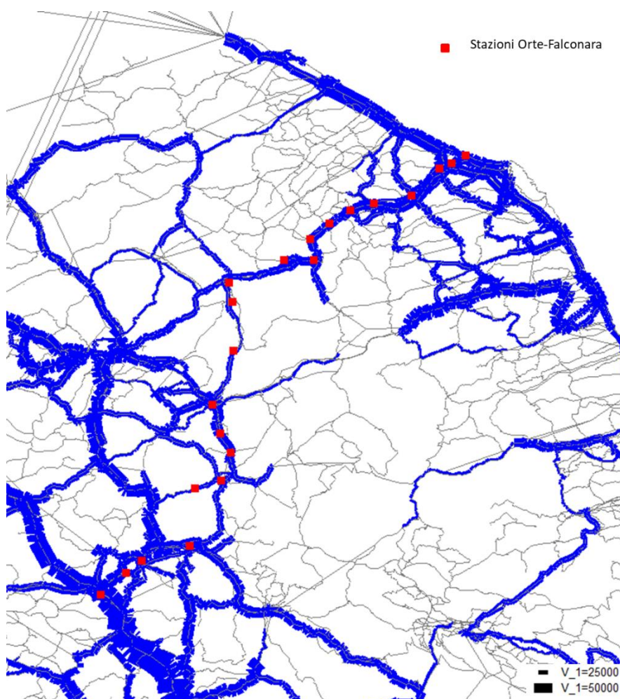
Figura 15 - Flussogrammi auto (veicoli/g), scenario riferimento 2026
