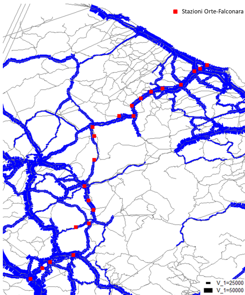
Figura 11 - Flussogrammi relativi al trasporto privato (veicoli/g), scenario 2019
