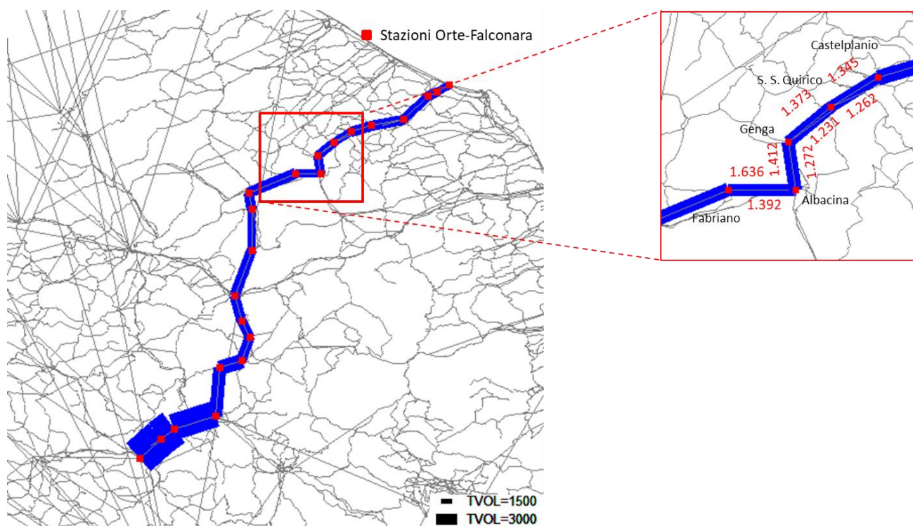
Figura 17 - Flussogrammi trasporto ferroviario (pax/g) linea Orte-Falconara, scenario di riferimento 2026
