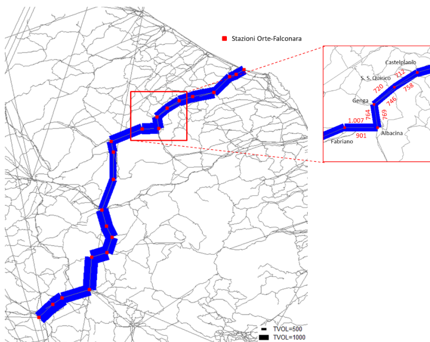
Figura 12 - Flussogramma del trasporto ferroviario (passenger/g), direttrice di progetto Orte-Falconara con focus sulle tratte di progetto, scenario 2019
