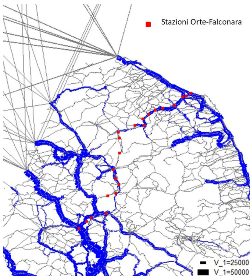
Figura 20 - Flussogrammi auto (veicoli/g), scenario progetto 2032
