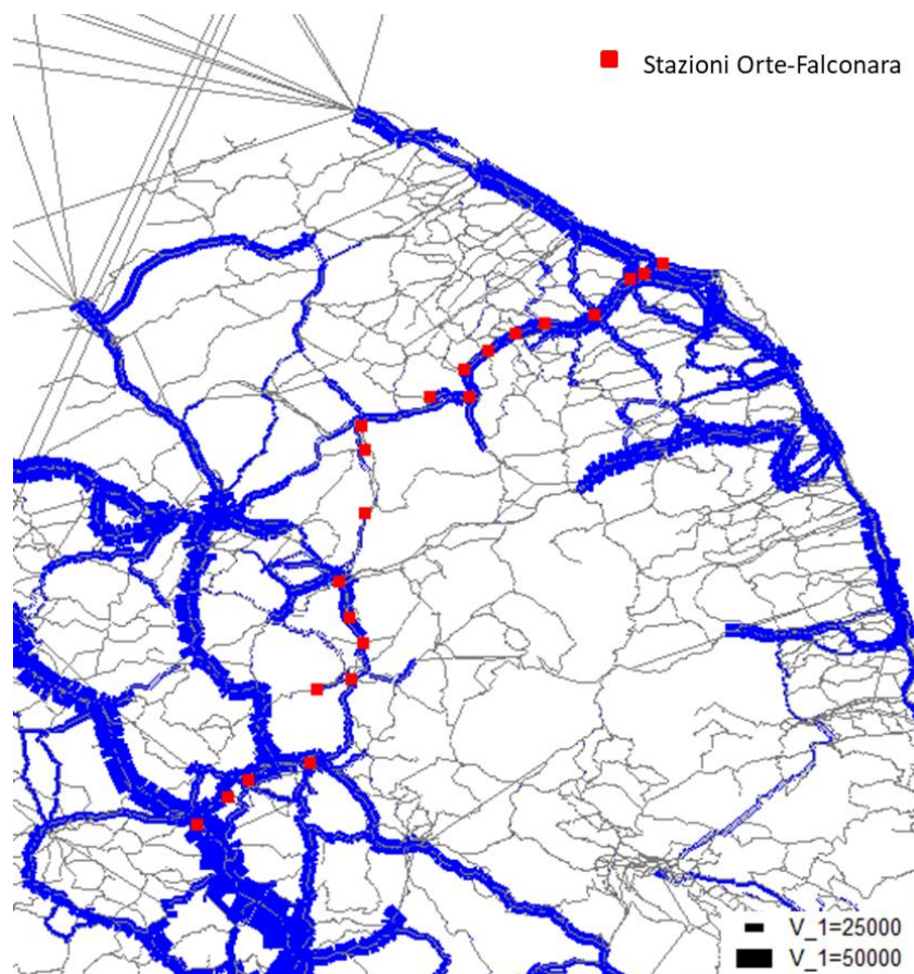
Figura 23 - Flussogrammi auto (veicoli/g), scenario riferimento 2035
