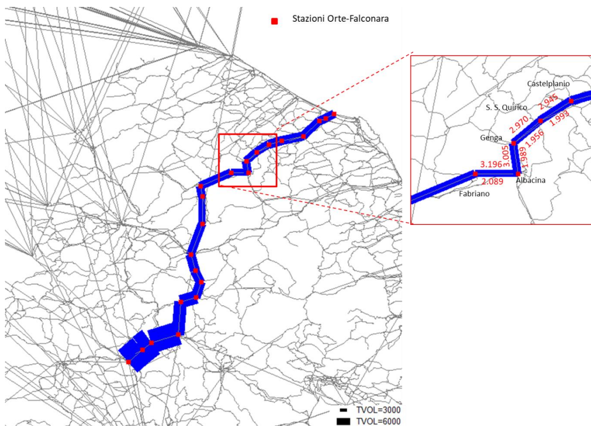
Figura 34 - Flussogrammi trasporto ferroviario (pax/g) linea Orte-Falconara, scenario di progetto 2064
