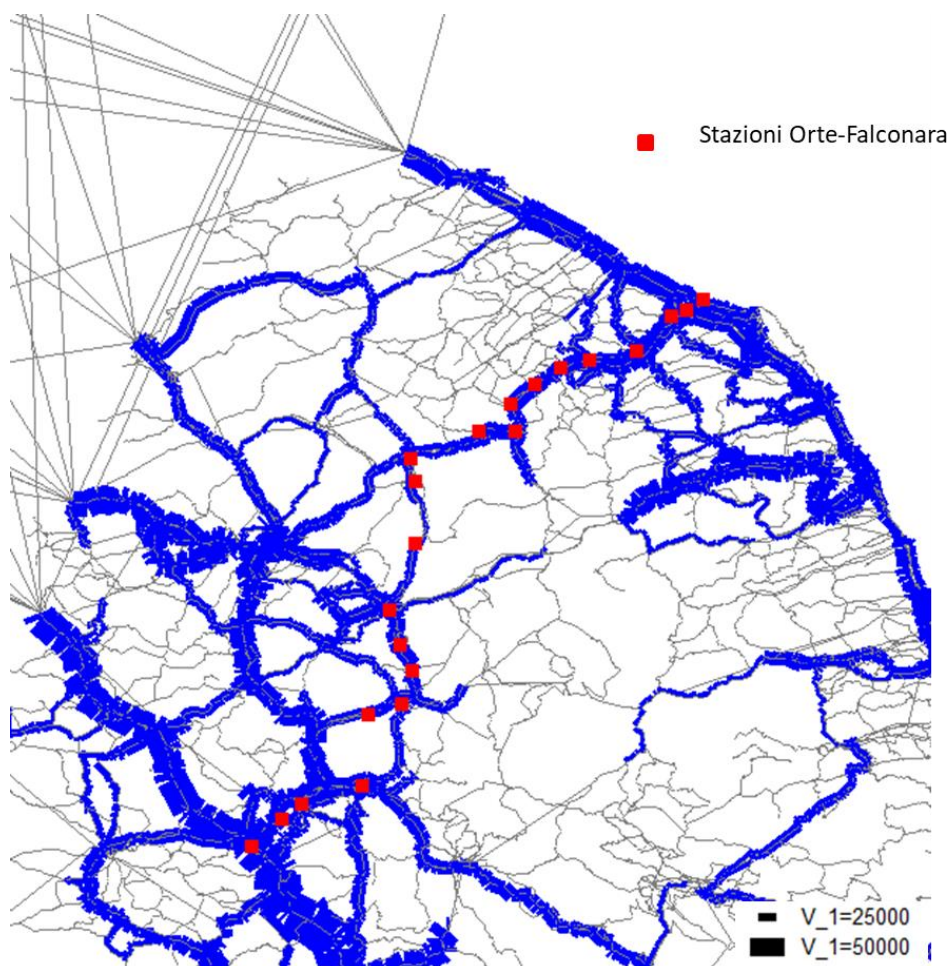
Figura 32 - Flussogrammi auto (veicoli/g), scenario progetto 2064
