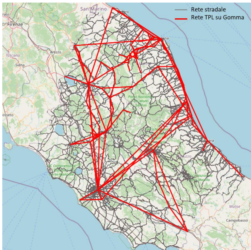
Figura 6 – Schema semplificato del grafo del trasporto pubblico su gomma dell'area di studio
