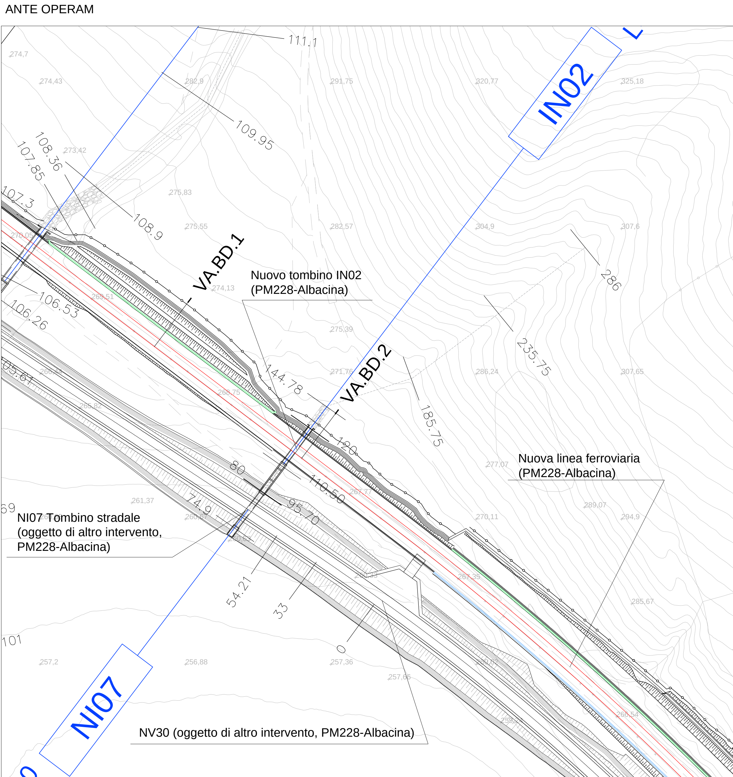
INQUADRAMENTO DEI CORSI D'ACQUA IN CORRISPONDENZA DEL TOMBINO IN03 - Scala 1:1000
