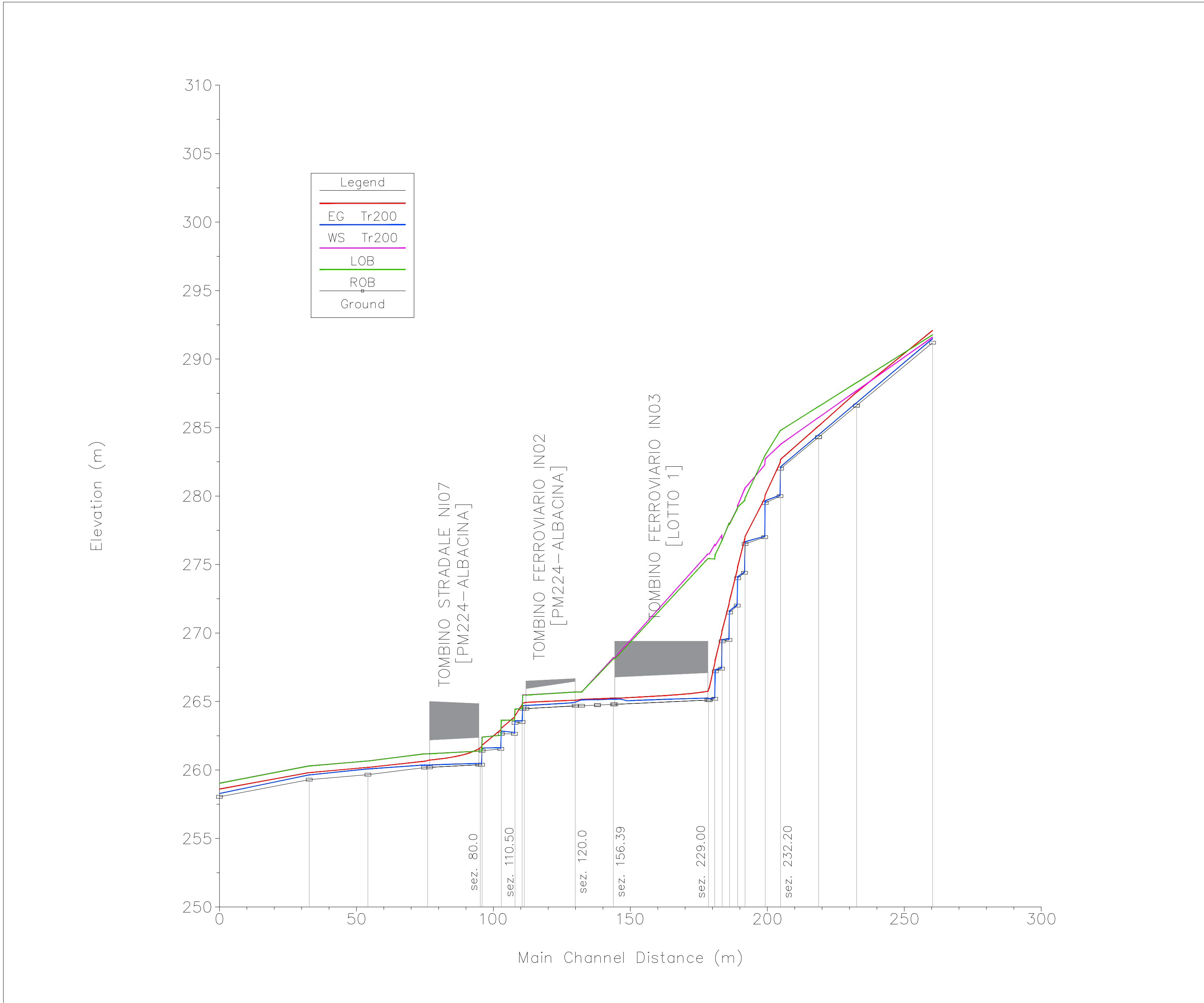
TOMBINO IN03: PROFILO RIGURGITO POST OPERAM - Scala 1:1000/1:200
