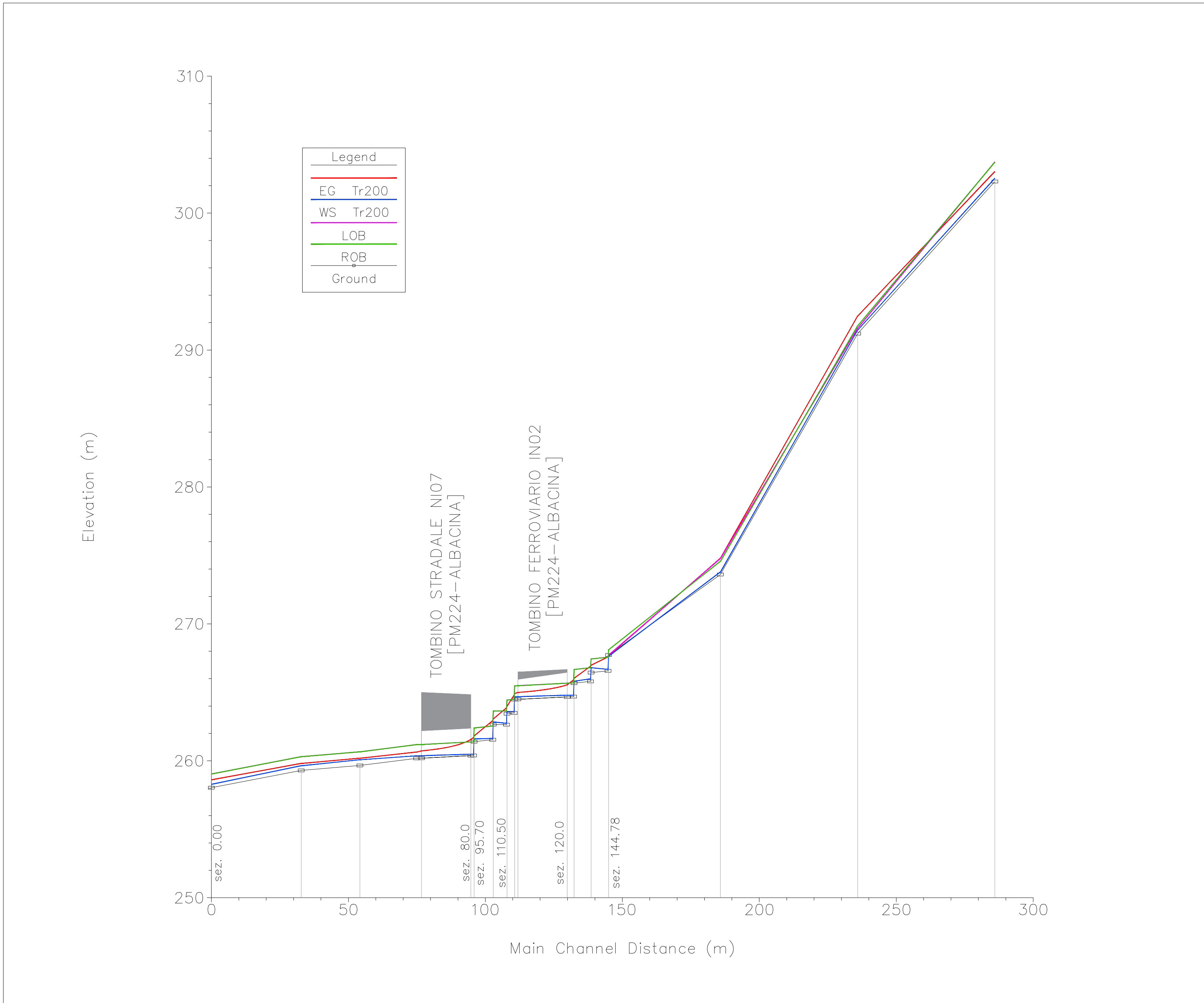
TOMBINO IN03: PROFILO RIGURGITO ANTE OPERAM - Scala 1:1000/1:200
