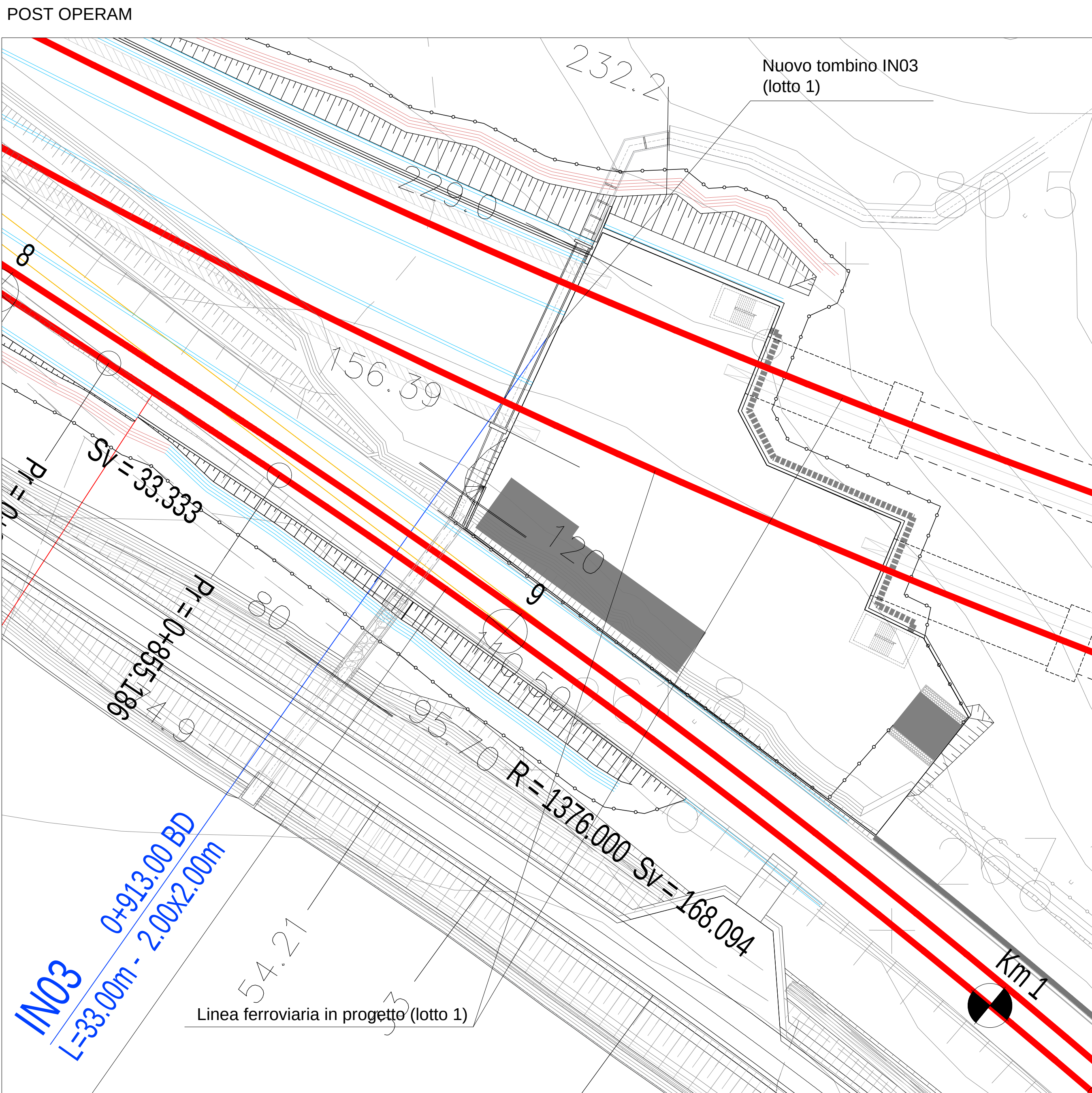
INQUADRAMENTO DEI CORSI D'ACQUA IN CORRISPONDENZA DEL TOMBINO IN03 - Scala 1:500
